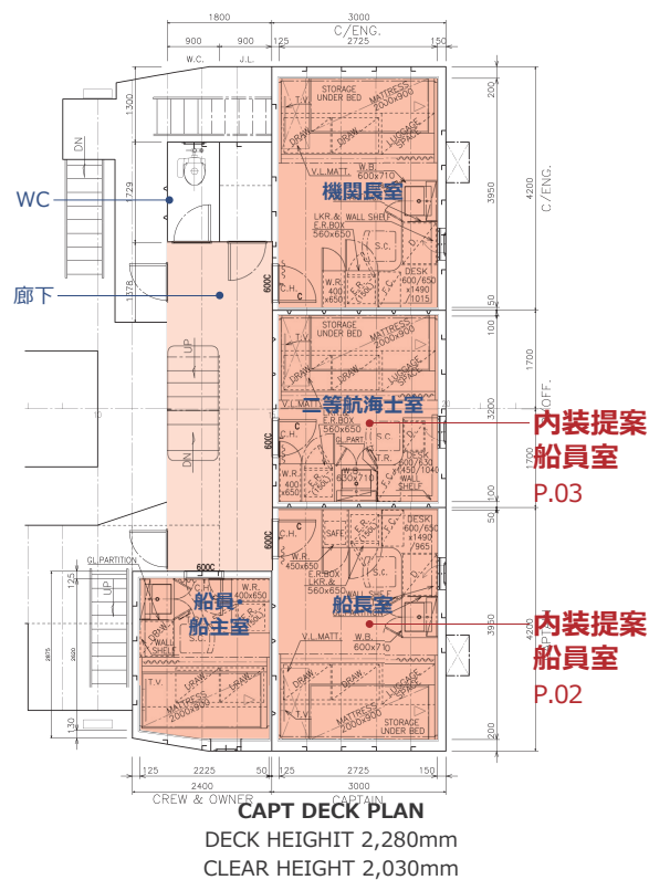
■平面図 S=1:100
