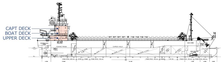
■一般配置図 S=1:600
